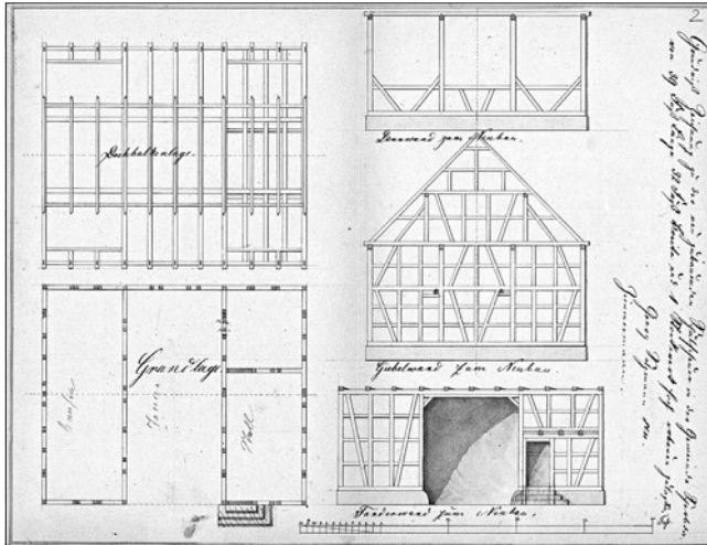
„Grundriß Zeichnung zu der neu zubauenden Schulscheune in der Gemeinde Scherbda. von 39 Fuß Länge 32 Fuß Breite und 1 Stockwerk hoch erbauen zulaßen. Georg Salzmann sen. Zimmermann.“[17].
