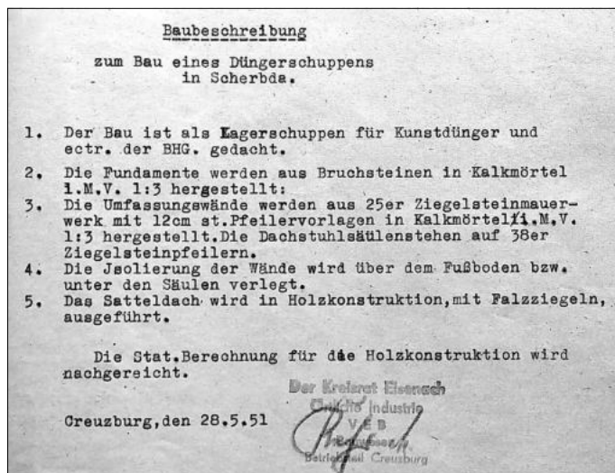
Baubeschreibung zum Bau eines Düngerschuppens für die VdgB-BHG in Scherbda[14].
