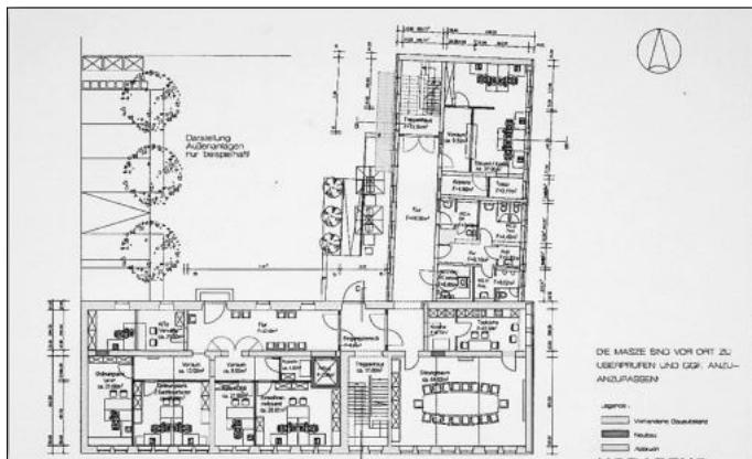
Planzeichnung des Erdgeschosses
