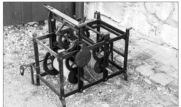
Das aus dem Jahr 1891 stammende Uhrwerk der Kirchturmuhre vor dem Wiedereinbau[8].
